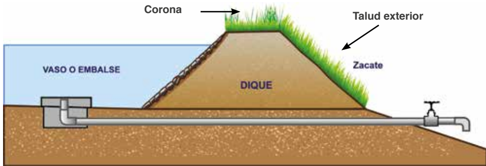
Ilustración 5: Talud exterior y corona protegidos con zacate. Fuente: CATIE.
