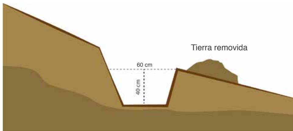
Figura 3. Excavación de acequias o zanjas a nivel o desnivel. Fuente: CATIE.
