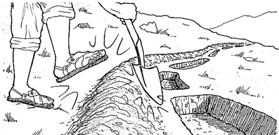
Figura 5. Acequia colectora de agua con barrera muerta de tierra. La tierra se compacta para que no caiga en la acequia. Fuente: JALDA 2003.
